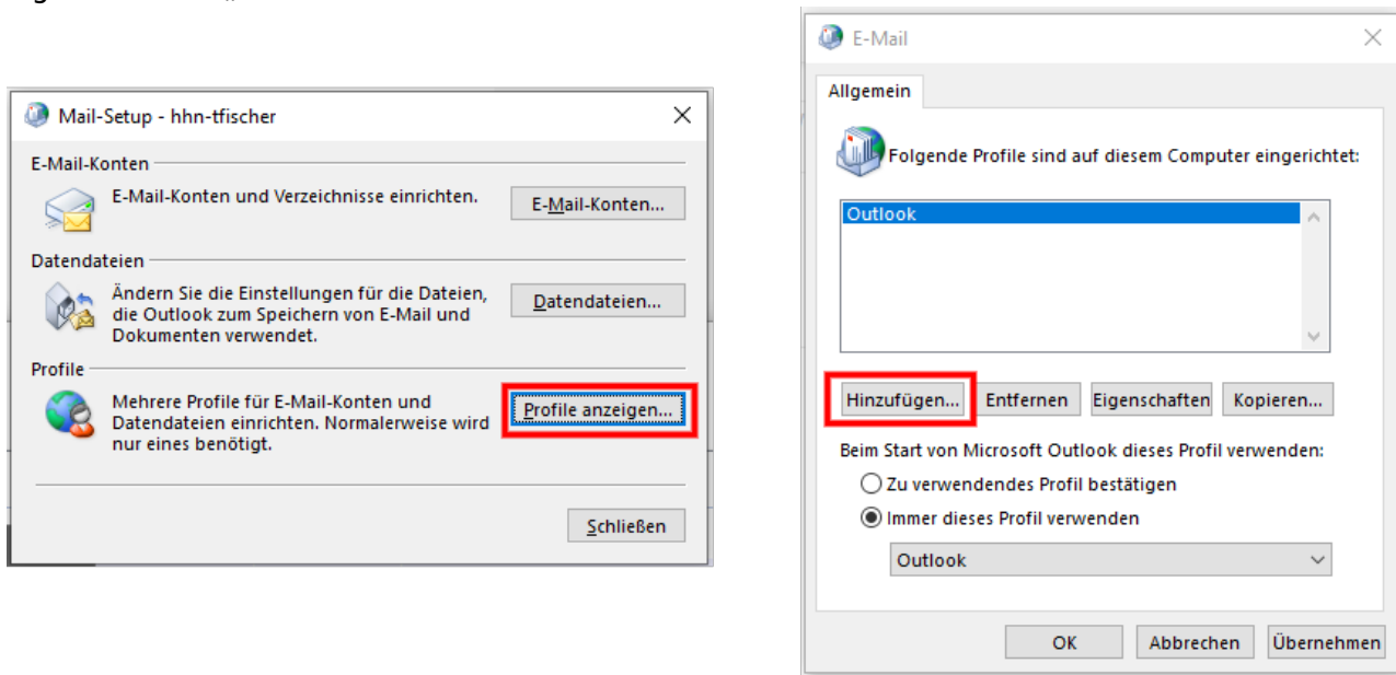
Fig. 1: Fenster „E-Mail“
