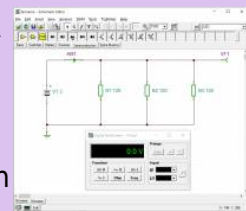
Fig. ##: Parallelschaltung 1
