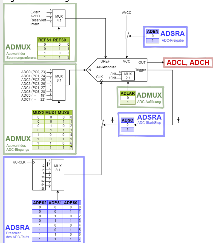
Fig. 1: Schaltung des AD-Wandlers im 328
