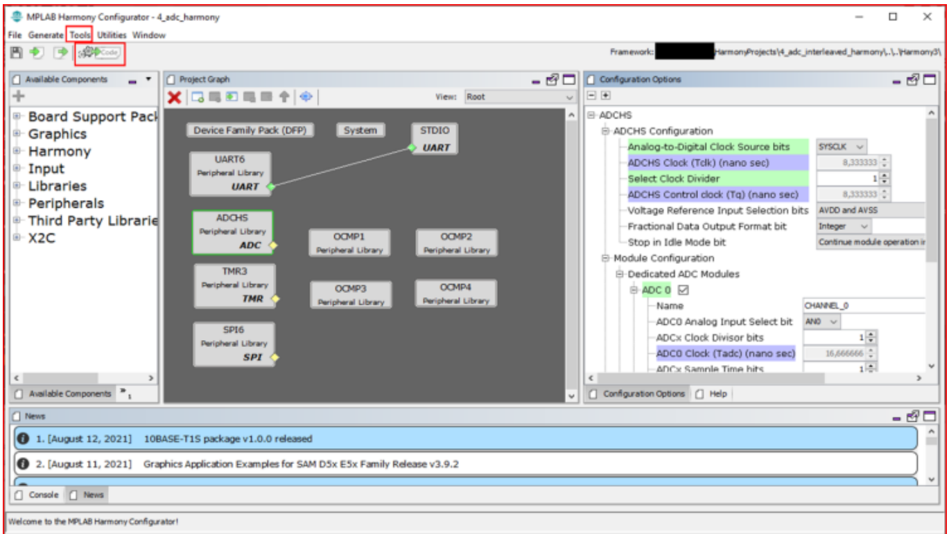
Fig. 25: Harmony Benutzeroberfläche
