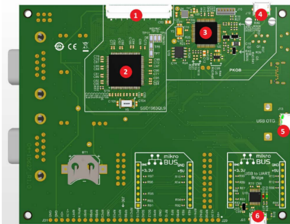
Abb. 15: Unterseite des Developmentboards DM320106
