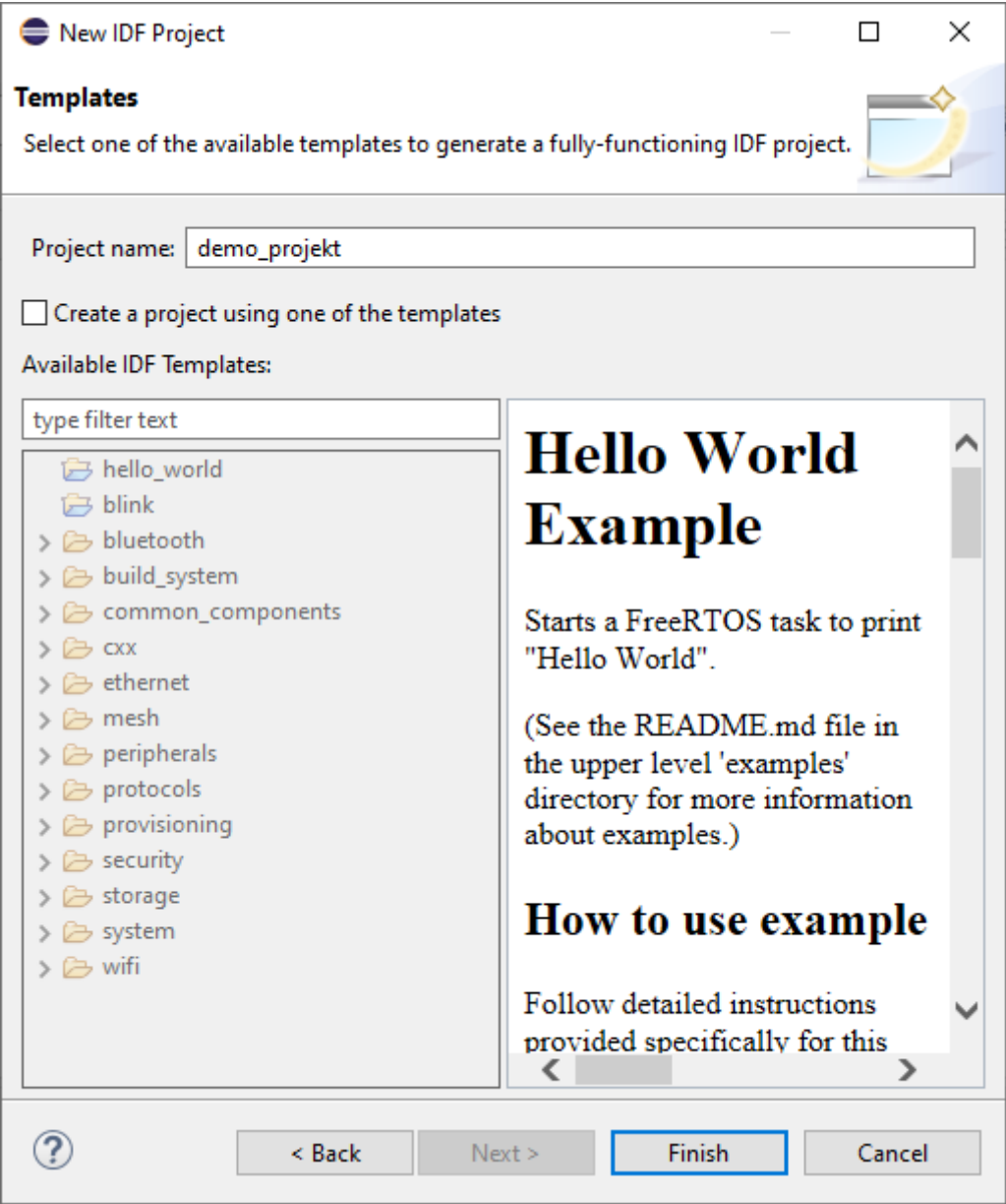
Abb. 45: Auswahlmöglichkeit leeres Projekt oder Beispielprojekt
