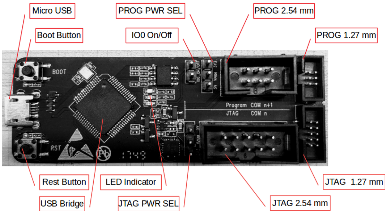
Abb. 20: ESP-Prog Programmer Platine für den ESP32 und ESP8266
