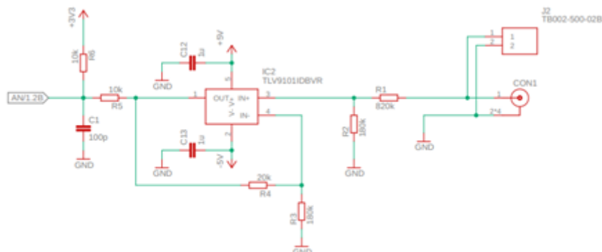
Abb. 5: Schaltplan der Messschaltung
