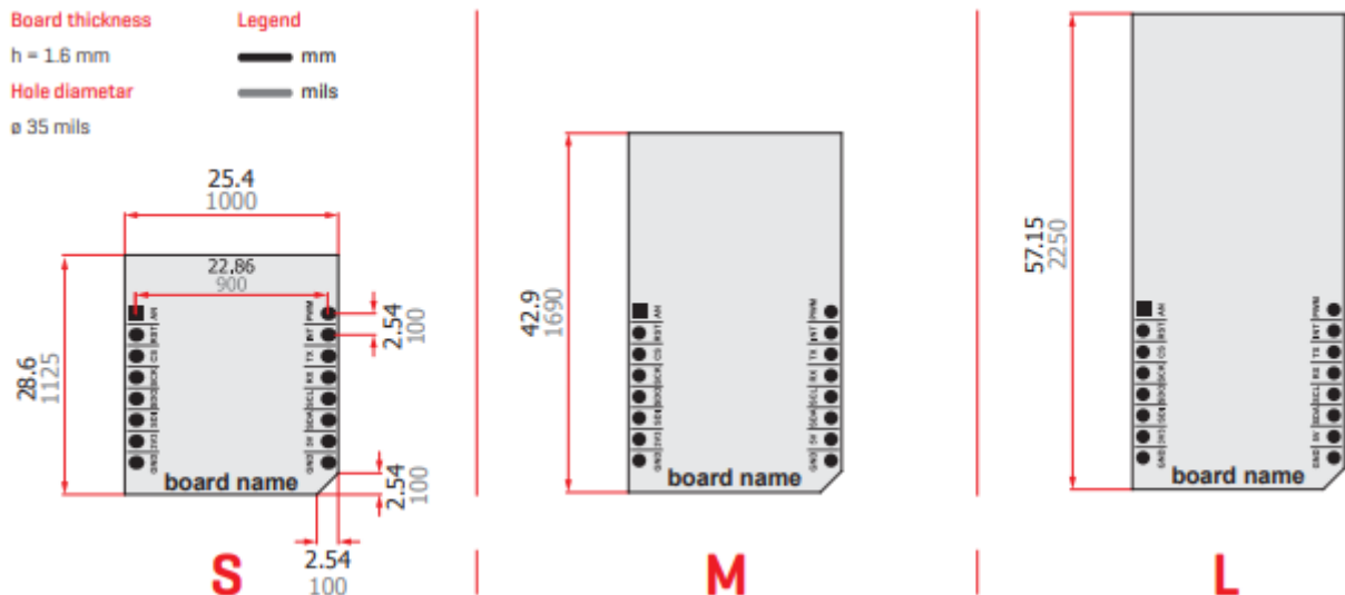
Abb. 16: Platinengrößen nach mikroBUS™ Standard
