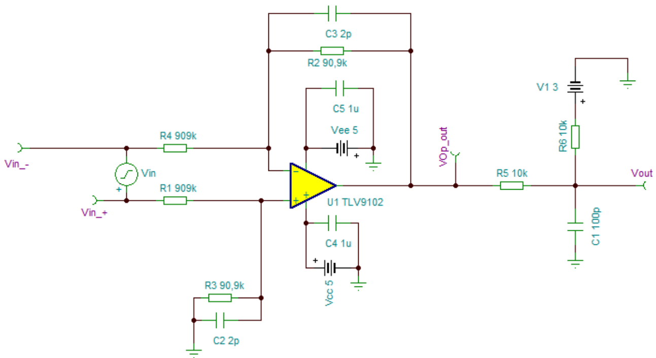
Abb. 10: Simulation differentielle Messschaltung
