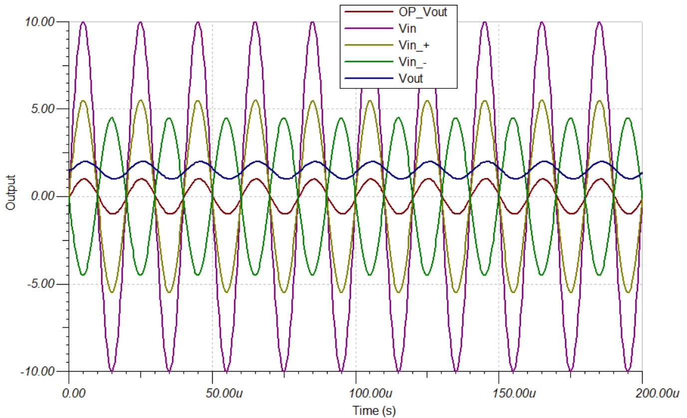
Abb. 11: Simulationsergebnis differentielle Messschaltung
