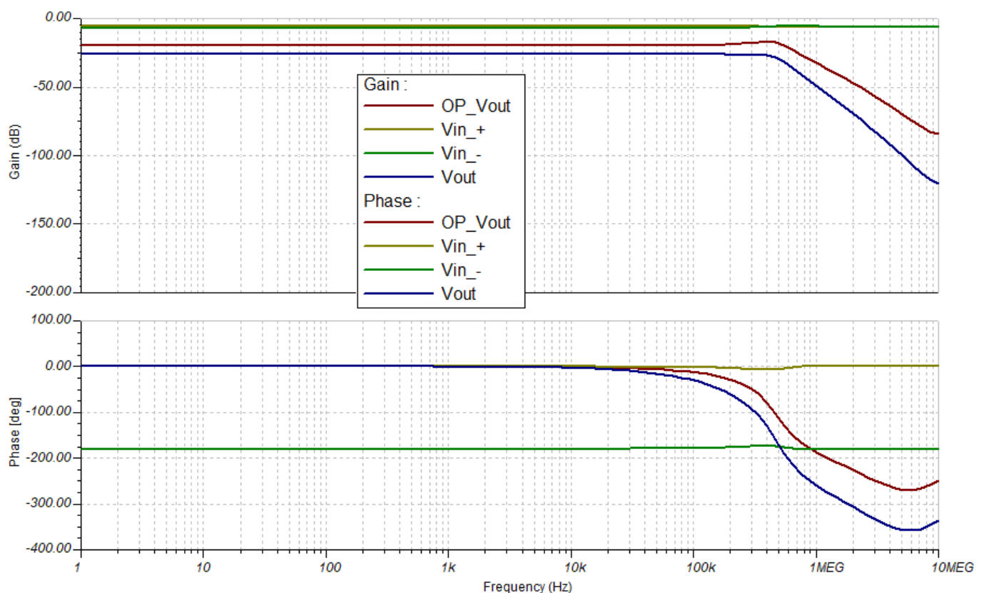
Abb. 12: Frequenz- und Phasengang differentielle Messschaltung
