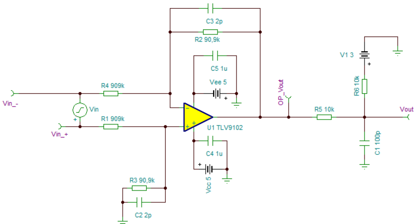
Abb. 7: Simulation der Messschaltung
