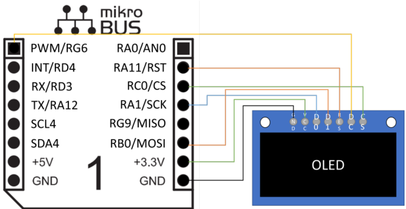
Abb. 32: Anschluss OLED
