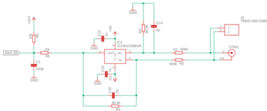
Abb. 6: Schaltplan der differentiellen Messschaltung
