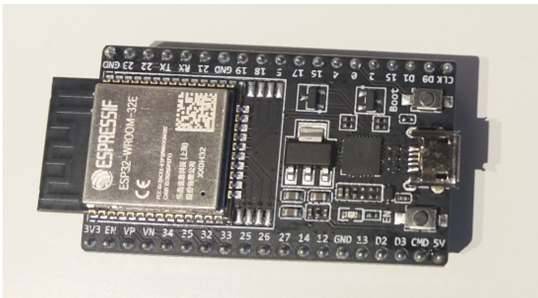
Abb. 50: Zur Programmierung der Demoprogramme verwendetes ESP32-DevKitC V4 Testkit
