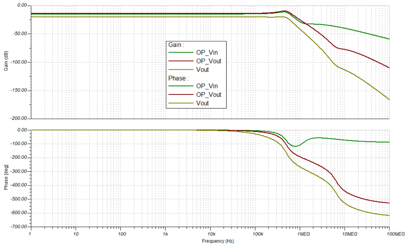
Abb. 9: Frequenz- und Phasengang Messschaltung
