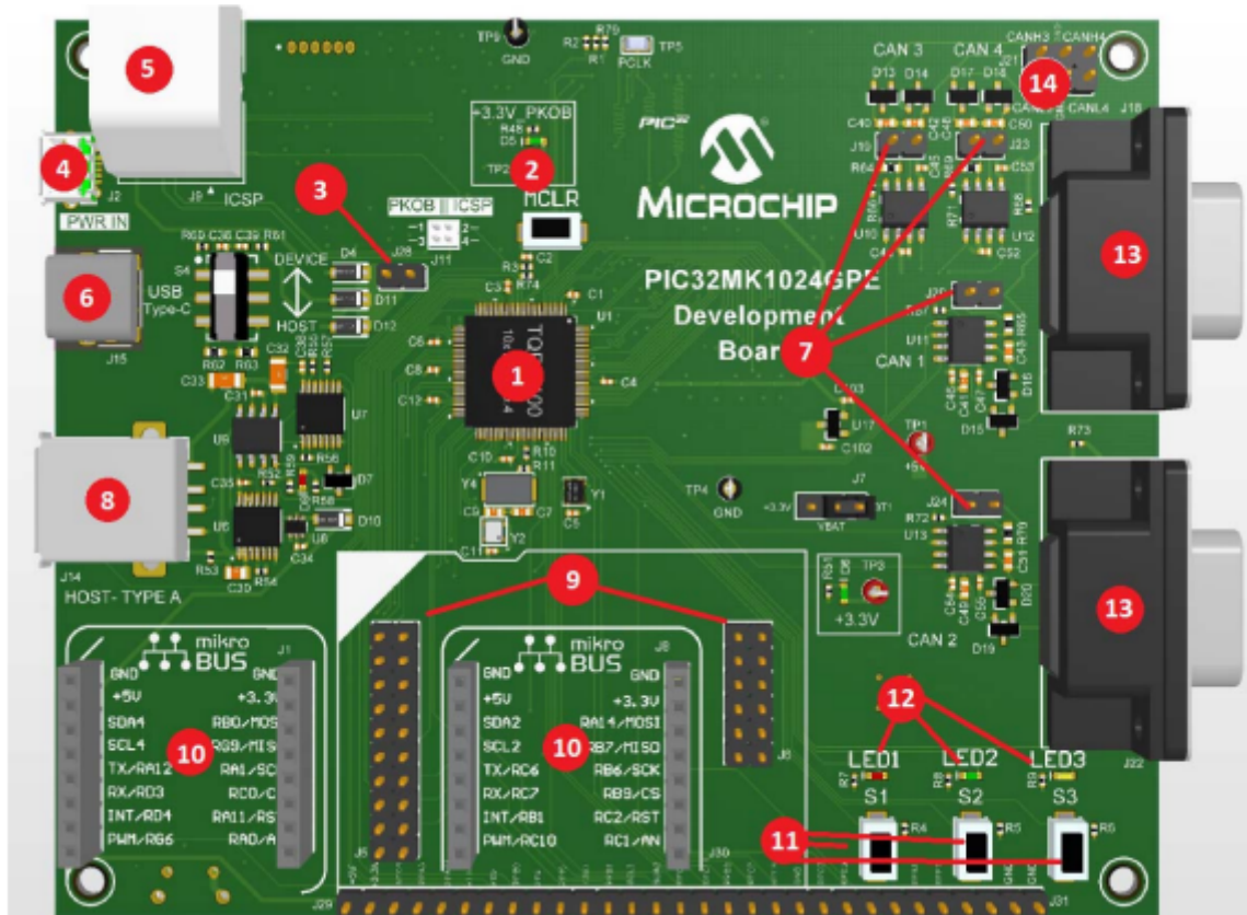
Abb. 14: Oberseite des Developmentboards DM320106
