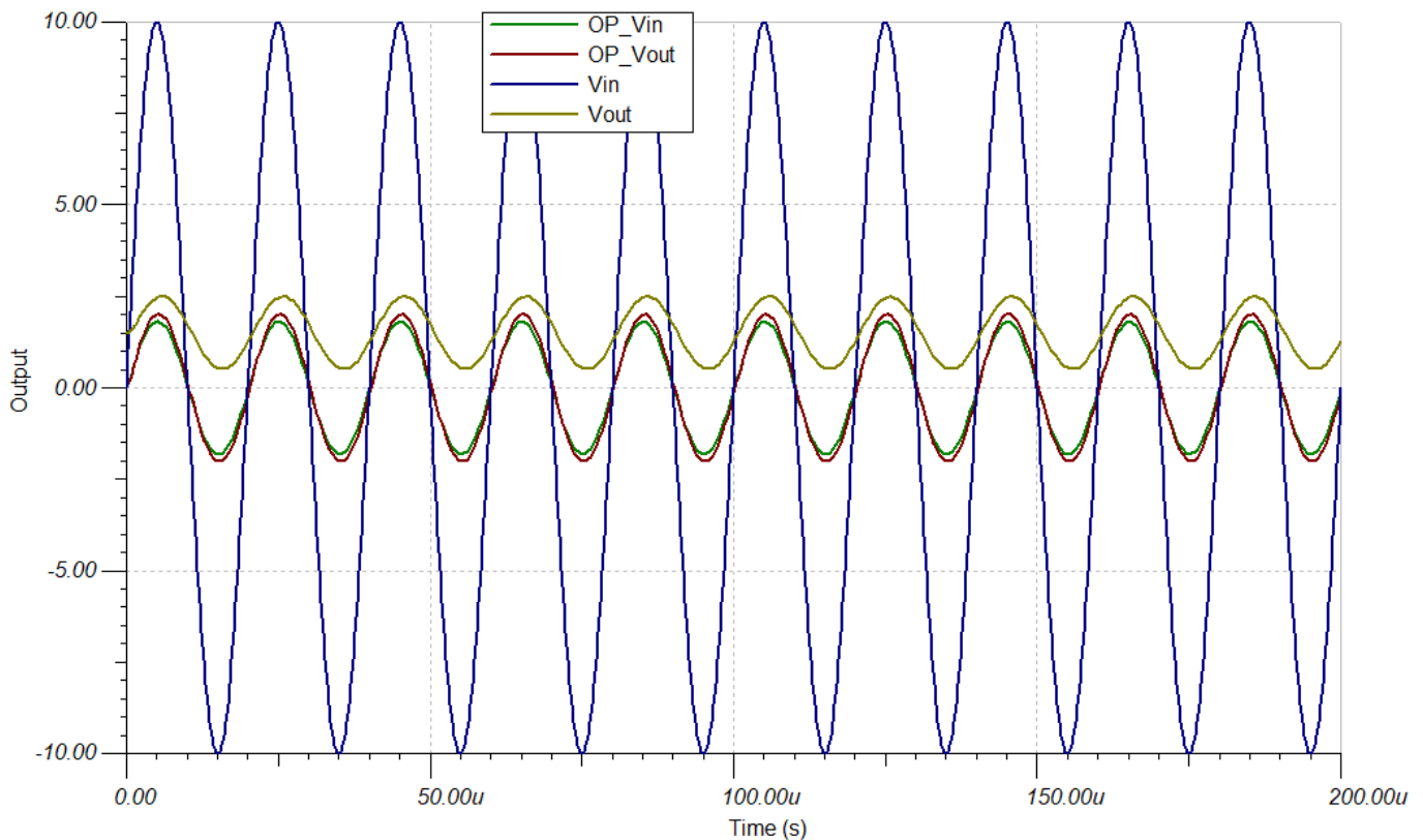
Abb. 8: Simulationsergebnis Messschaltung
