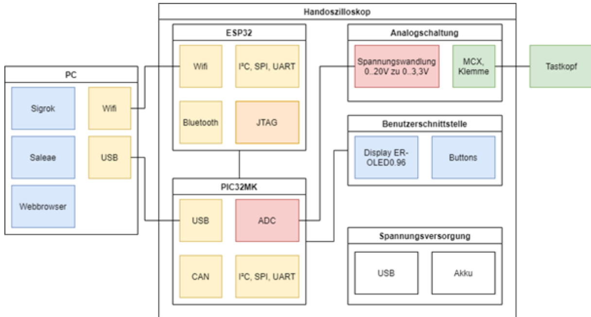
Abb. 1: Handoszilloskop Systemübersicht
