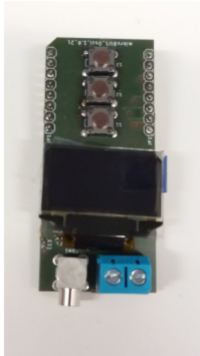
Abb. 19: Bestückte mikroBUS Oszilloskop Platine
