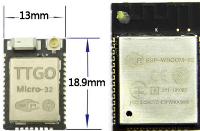
Abb. 4: Vergleich TTGO Micro32 und ESP32 WROOM Quelle Abbildung 4: 16)
