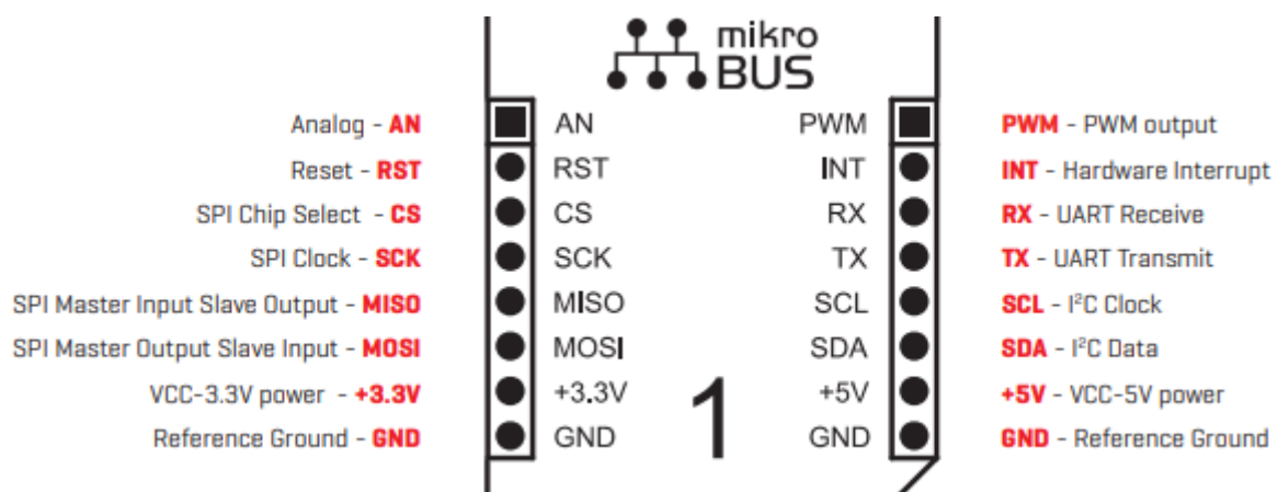
Abb. 17: Pinbelegung eines Boards nach mikroBUS™ Standard
